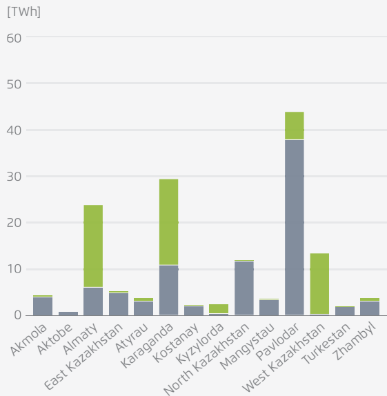
OPT^2 scenario
