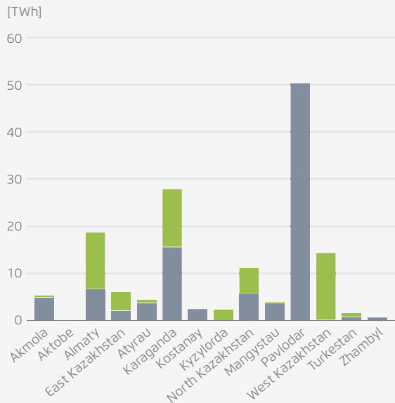
BAU scenario
