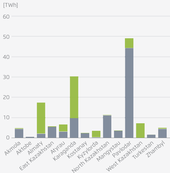
OPT scenario
