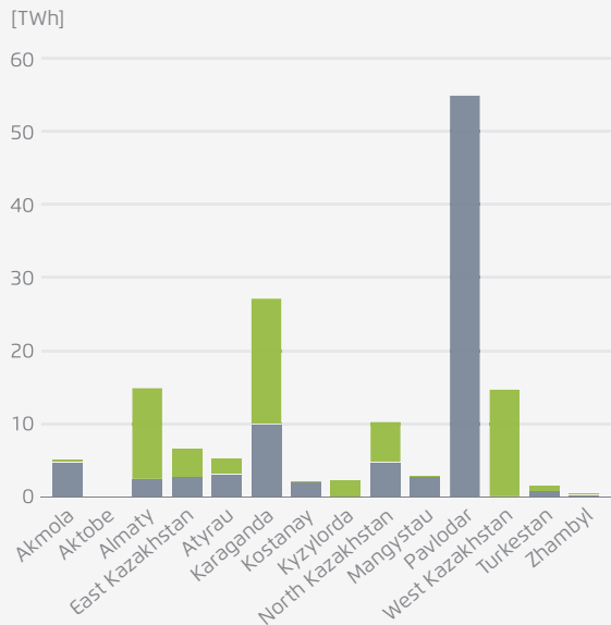
iBAU scenario
